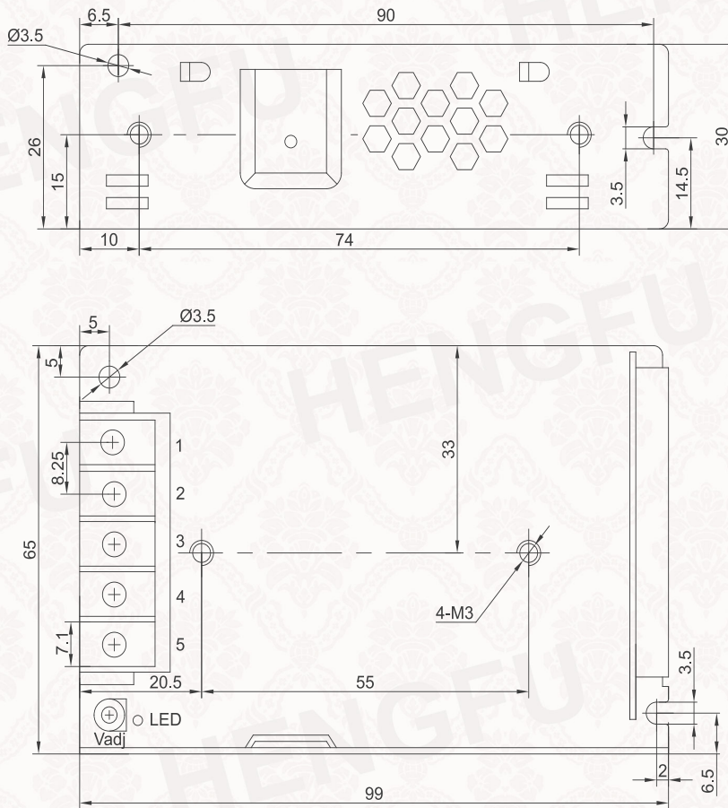
机壳 Frame
